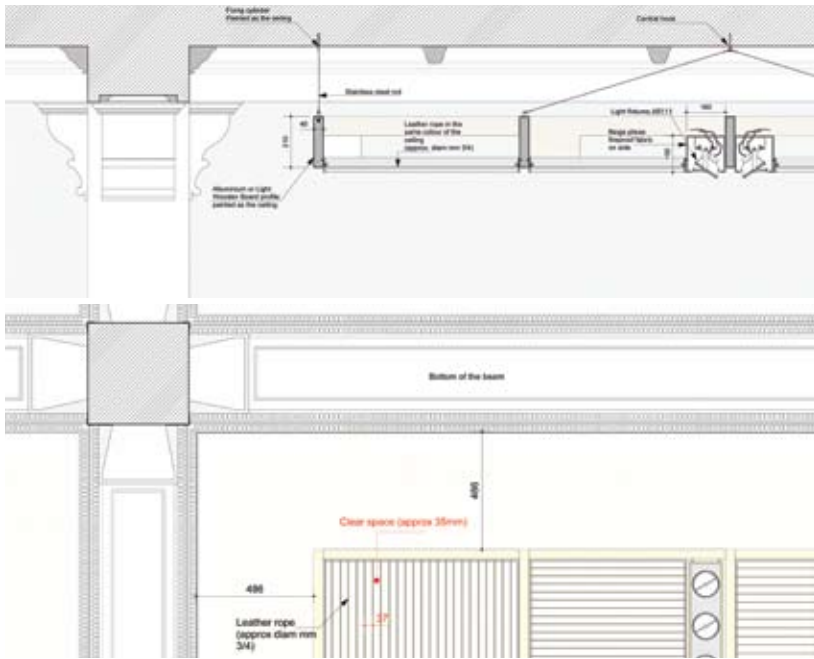
Studio tecnico dei "light rafts" / "Light rafts" technical study
