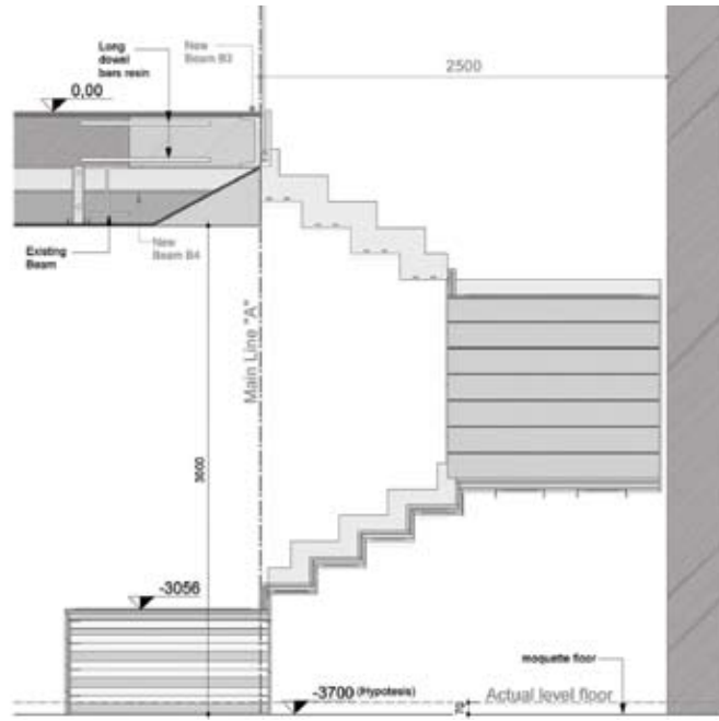
Studio tecnico della scala / Staircase technical study
