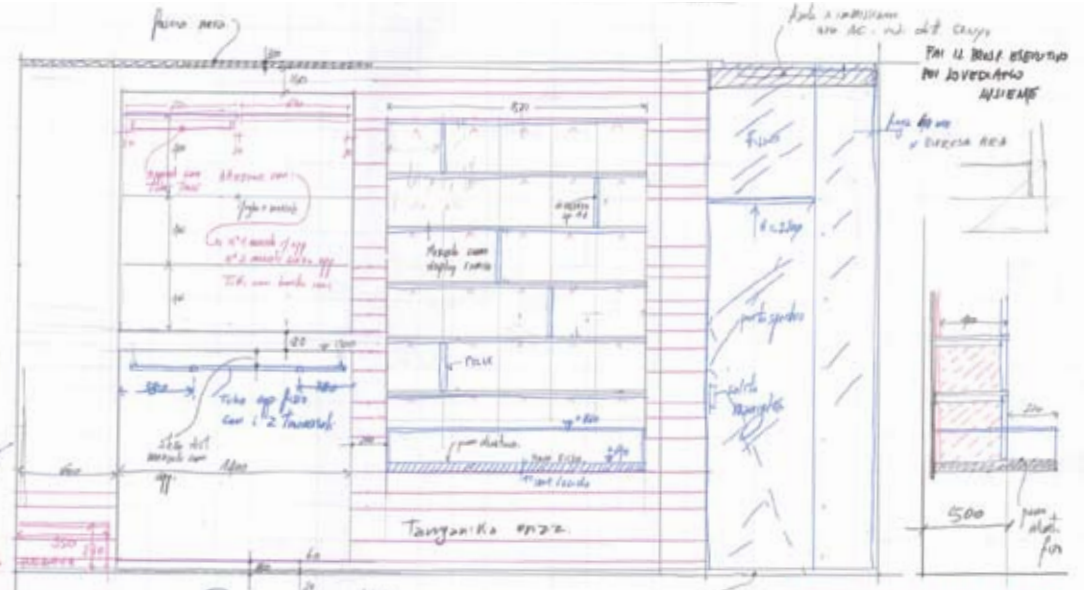
Sistema espositivo, dettaglio e studio progettuale / Display system, detail and concept sketch
