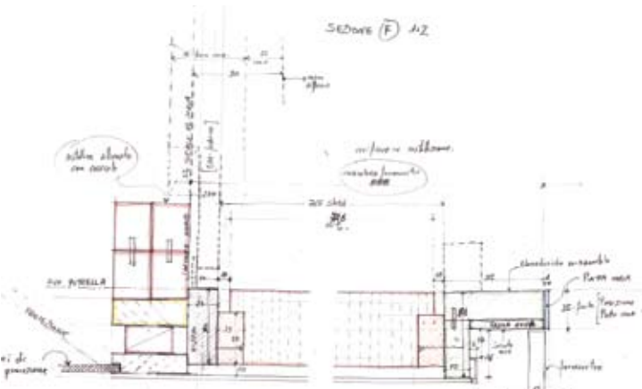
Studio esecutivo della parete riflettente / Reflecting wall - executive sketch
